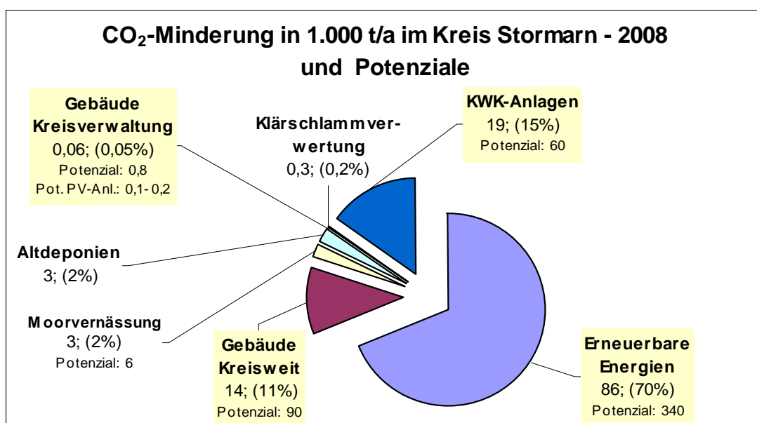
Abb. 2: Klimaschutzeffekte und Potenziale ausgewählter Handlungsfelder
